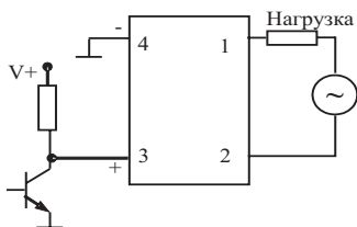
NPN, нормально-замкнутый
