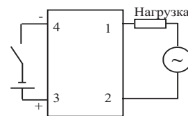
Реле, нормально-разомкнутый
