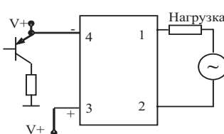
PNP, нормально-замкнутый
