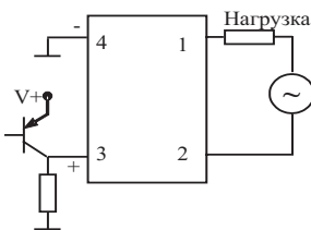
PNP, нормально-замкнутый
