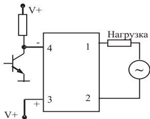
NPN, нормально-замкнутый
