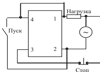
Схема с самоблокировкой (AC-AC)
