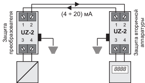
Схема элэлектрических присоединений
