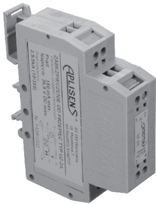
Вариант на рейке TS-35 и TS-32
