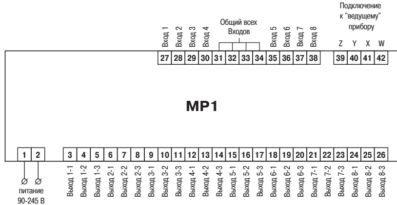
Рис. Б1. Схема расположения клемм MP1
