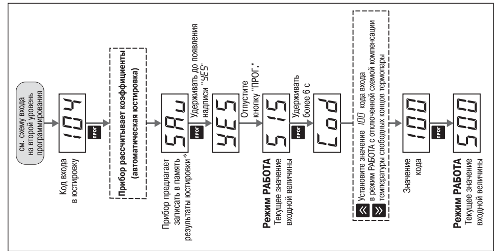
Схема П4.2. Последовательность действий при юстировке прибора с термопарой
